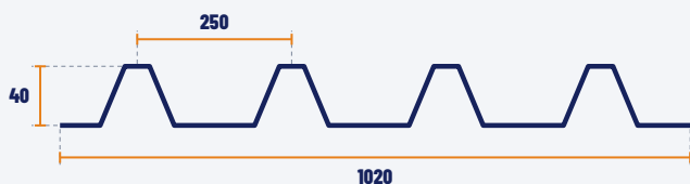
Poprečni presek TR 40 (šematski) · mere u mm
